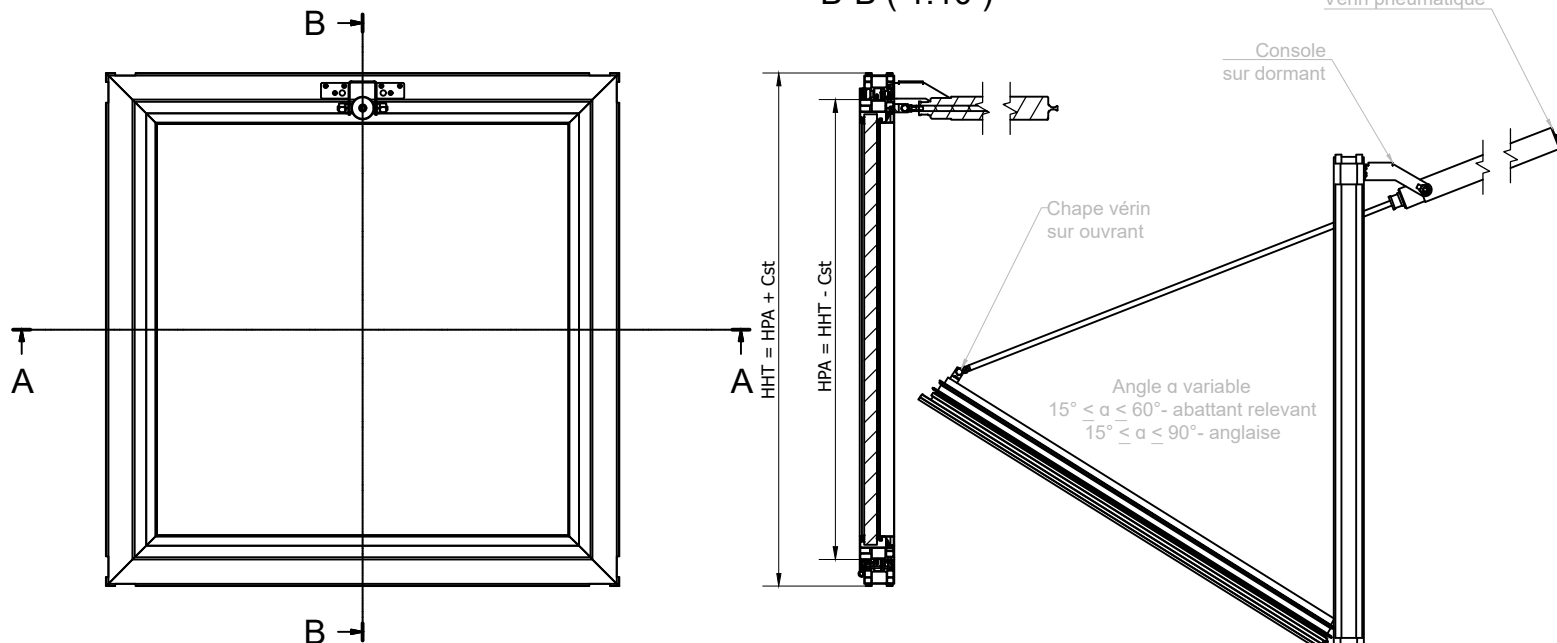
B-B ( 1:10 )
